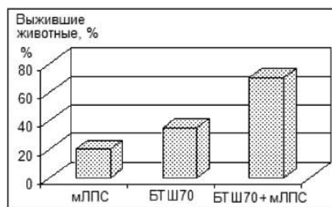
Рис. 2. Влияние экзогенного БТШ70 и мЛПС на выживаемость мышей при экспериментальном эндотоксическом шоке.
